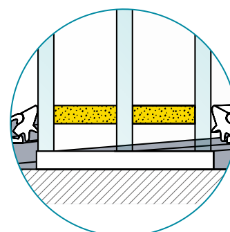
Dreifachverglasung mit zwei Kunststoff- Abstandhaltern
