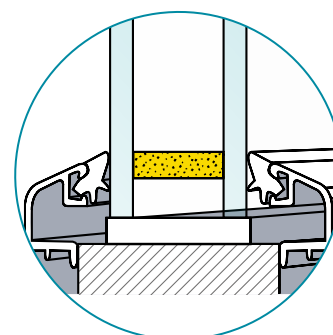
Kunststoff-Abstandhalter
