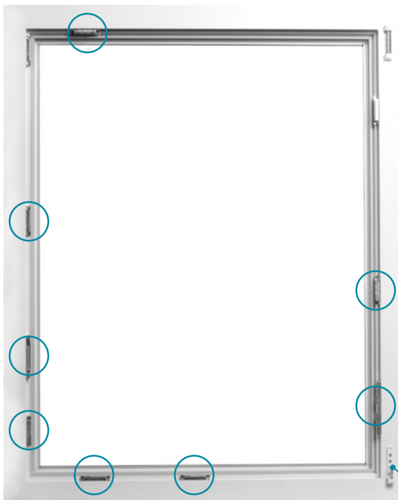
8 Sicherheitsschließteile pro Fenster (verhindern das Aushebeln)
